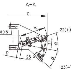
Чертеж 2 Реверсор
