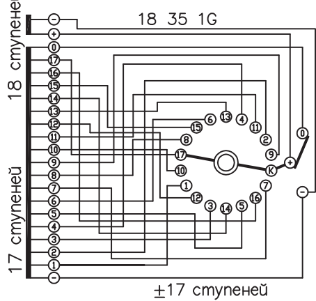
Схема 6б: Основные схема соединений
