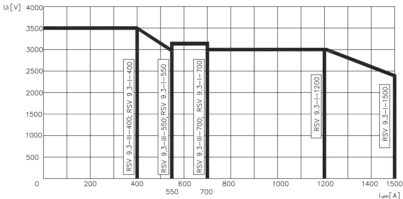
Схема 1: Номинальные переключающие способности (номинальный ток нагрузки I_u (A); номинальные ступенчатые напряжения U_i (V))
